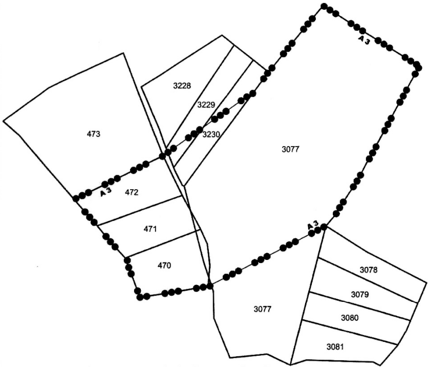
CANBAZ 3. DERECE ARKEOLOJİK SİT KÖŞE KOORDİNAT LİSTESİ
